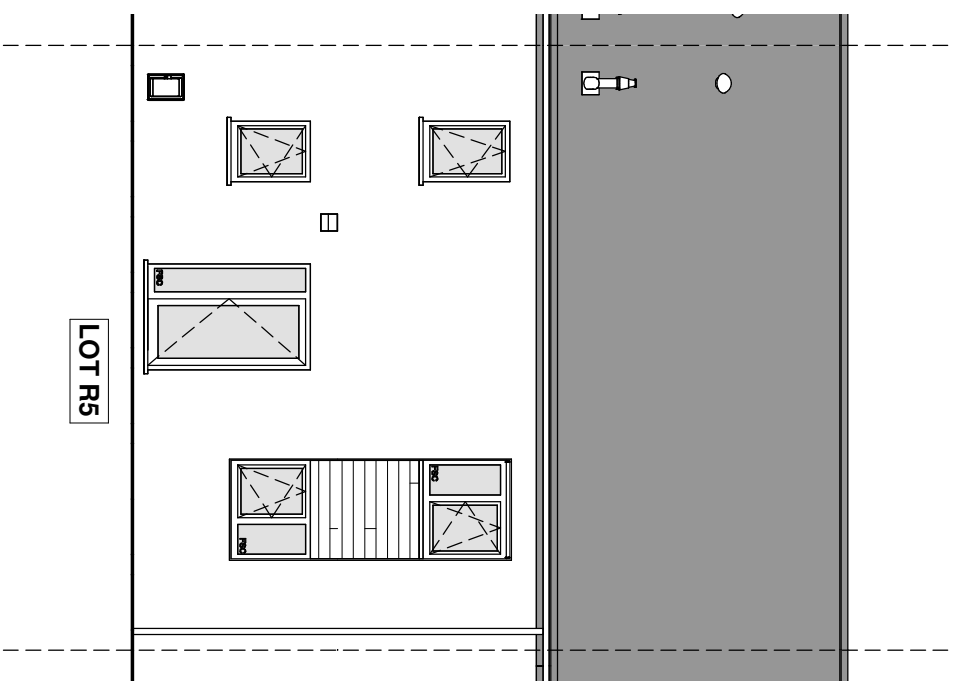
FACADE AVANT
